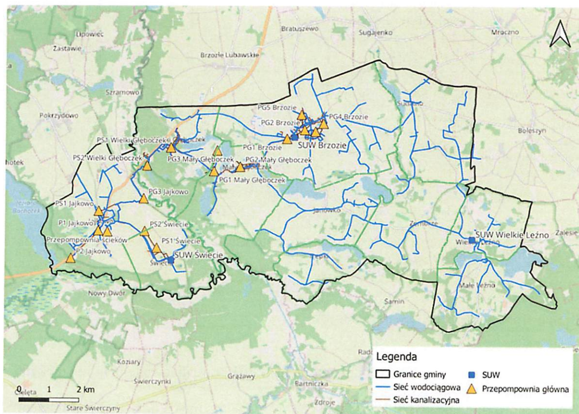
Rys. 1. Gmina Brzozie - sieci i obiekty wod-kan.
